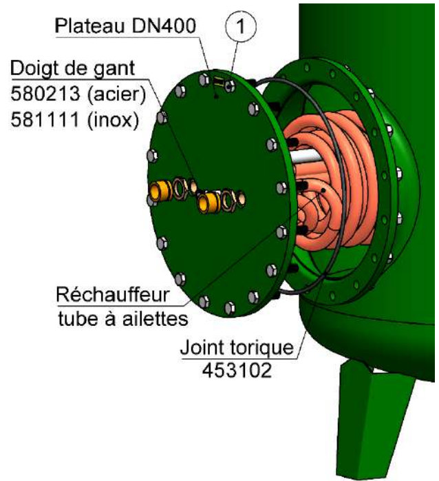
Réchauffeur 750L à 3000L
